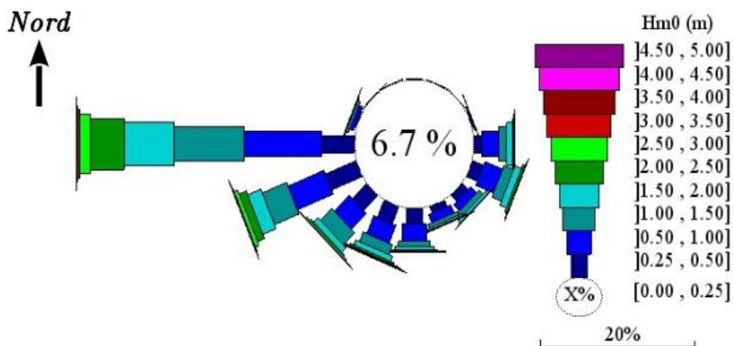
Figure 24 : climat rose des houles à la bouée houlographe de Porquerolles (CEREMA, 2016)
