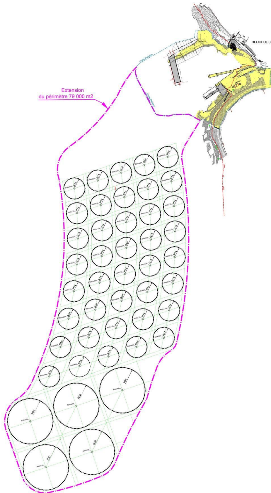
Figure 8 : Périmètre d'extension portuaire et plan d'organisation de la zone de mouillages
