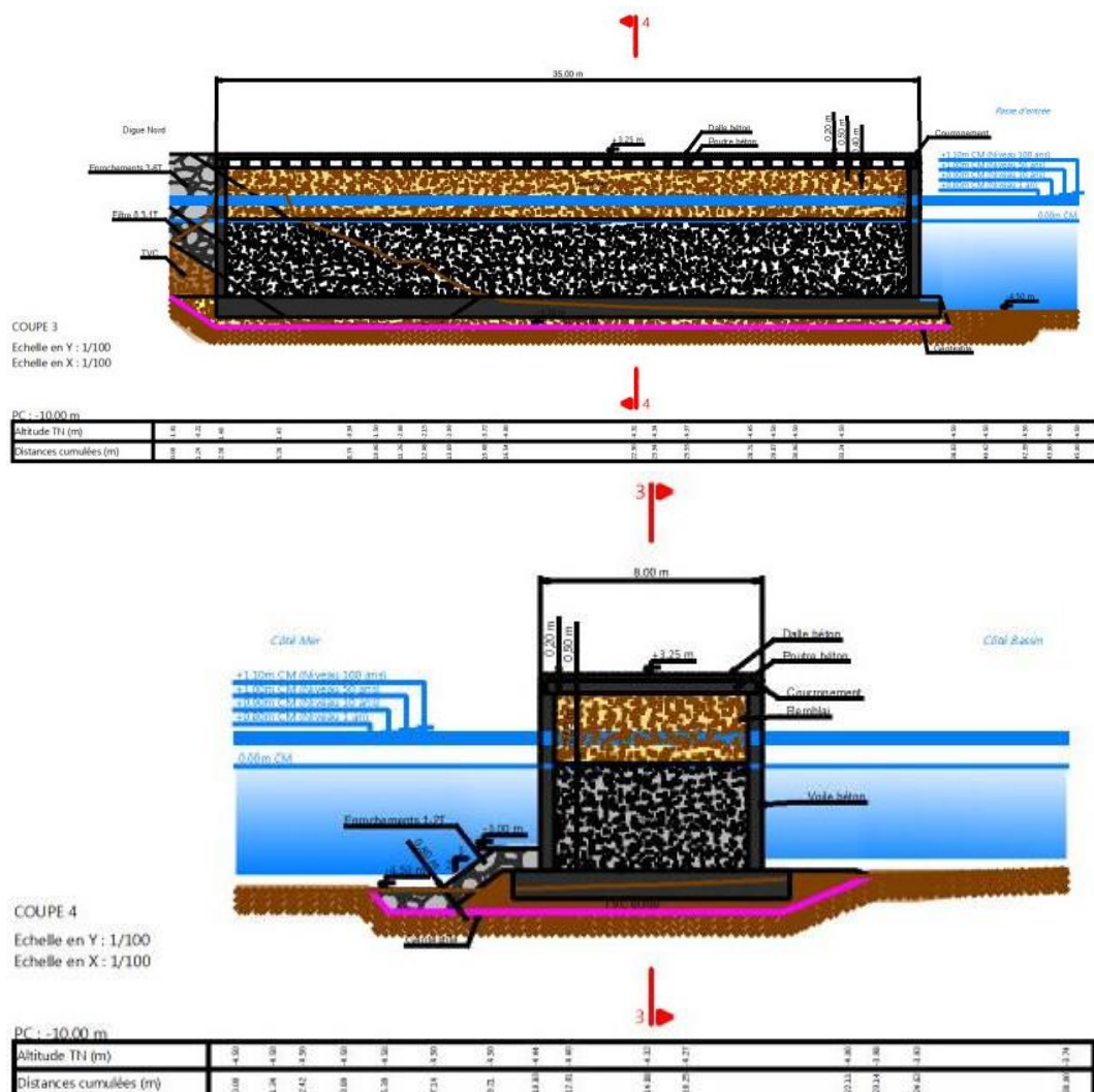
Figure 16 : Quai poids vertical - Coupes 3 et 4 de la Figure 14 p31
