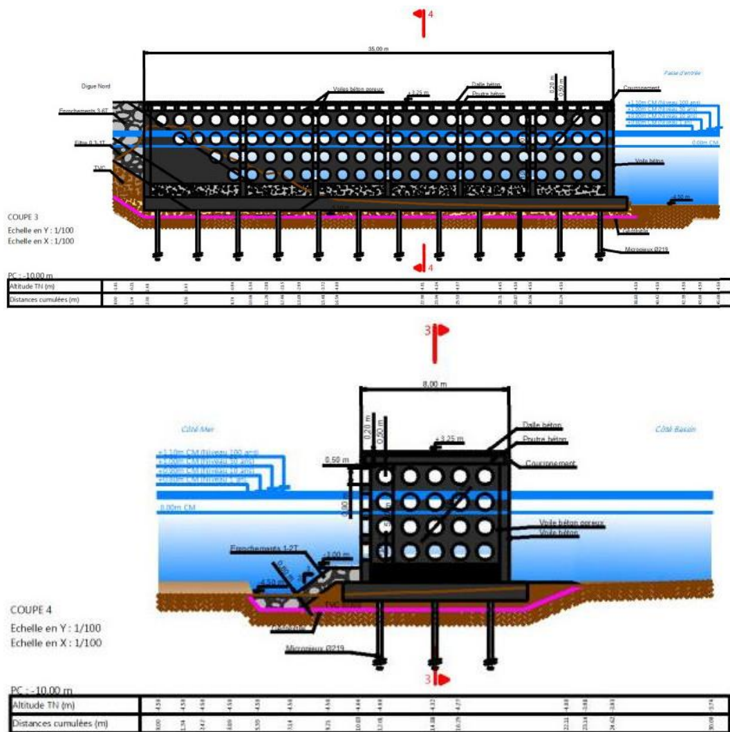
Figure 17 : Caisson amortissant de type Jarlan – Coupes 3 et 4 de la Figure 14 p31
