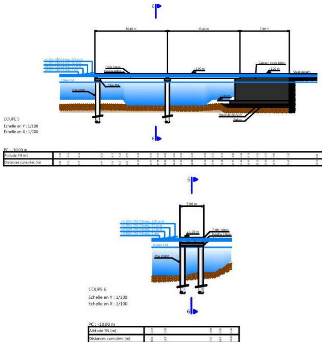
Figure 19 : Quai Ro-Ro- Coupes 5 et 6 de la Figure 14 p31
